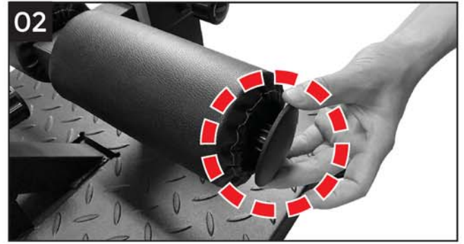
02 쿠션캡을 발걸이 쿠션에 조립하여 줍니다.
