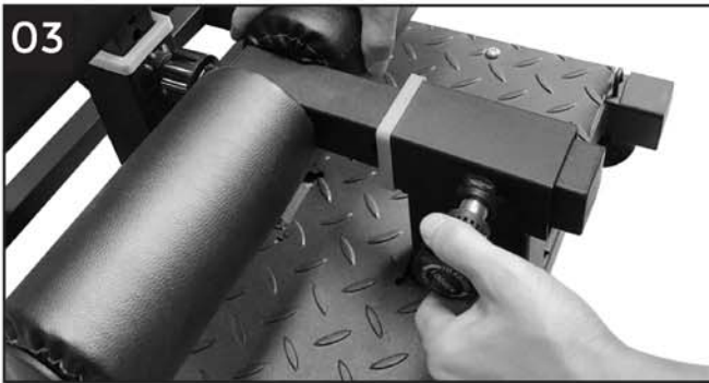
03 발걸이 지지대 고정볼트를 조립하여 줍니다.
